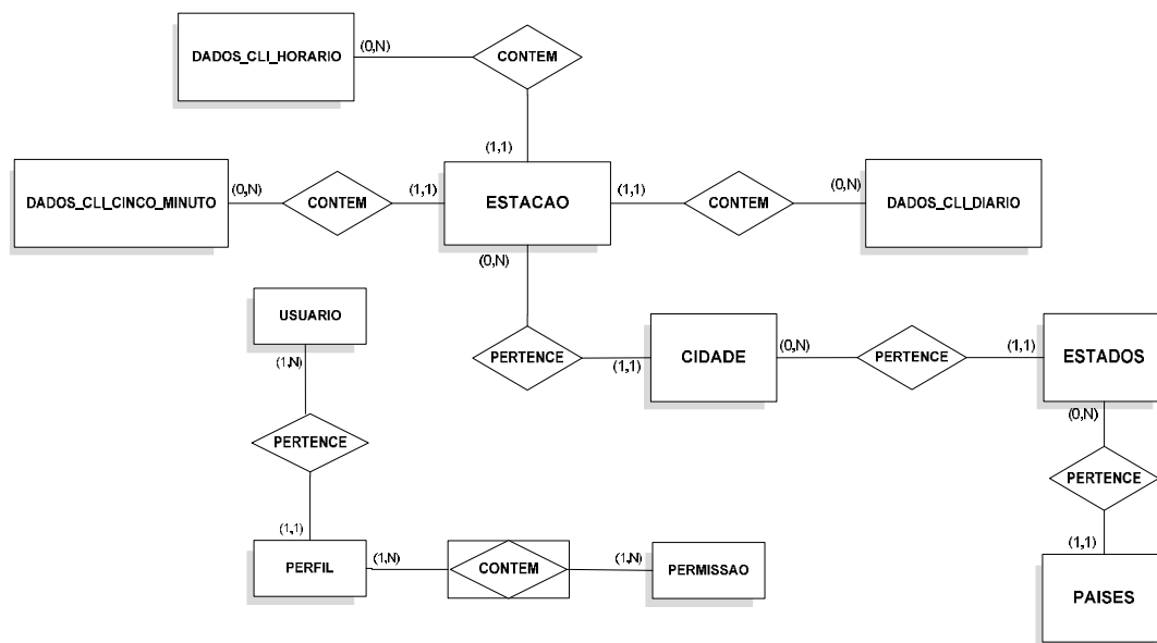
Figura 1. Diagrama de Entidades e Relacionamento.
