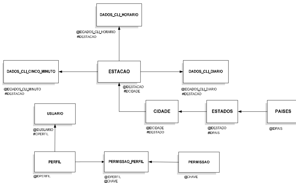
Figura 2. Diagrama de Estrutura de Dados.
